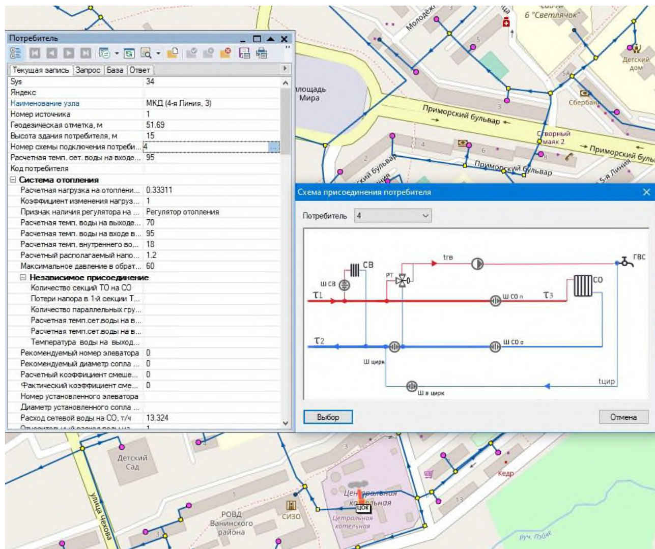
Рисунок 3.1.3-1. Графическое представление системы теплоснабжения рабочего поселка Ванино с привязкой к топографической основе поселка с полным топологическим описанием связности объектов.
