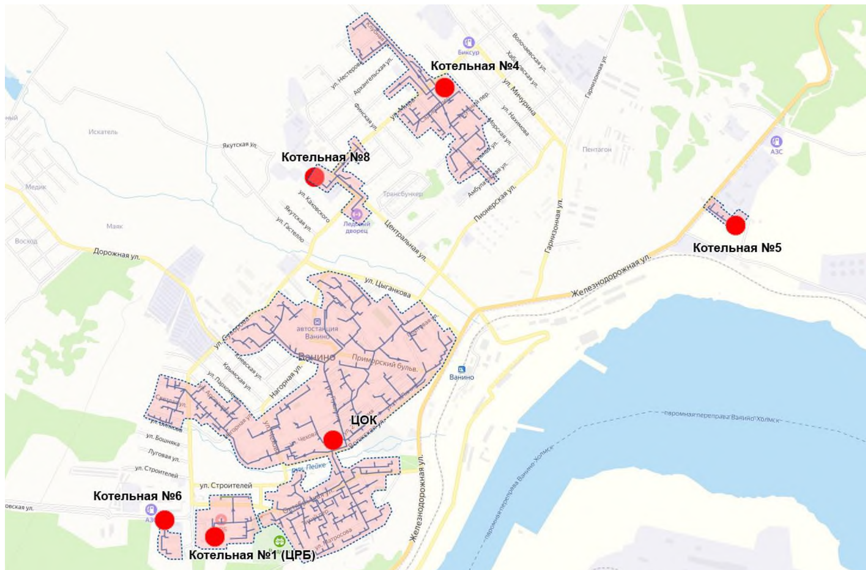
Рисунок 1.3-1 - Схема поселения, Городского поселения с указанием зон деятельности (эксплуатационной ответственности) теплоснабжающих и теплосетевых организаций
