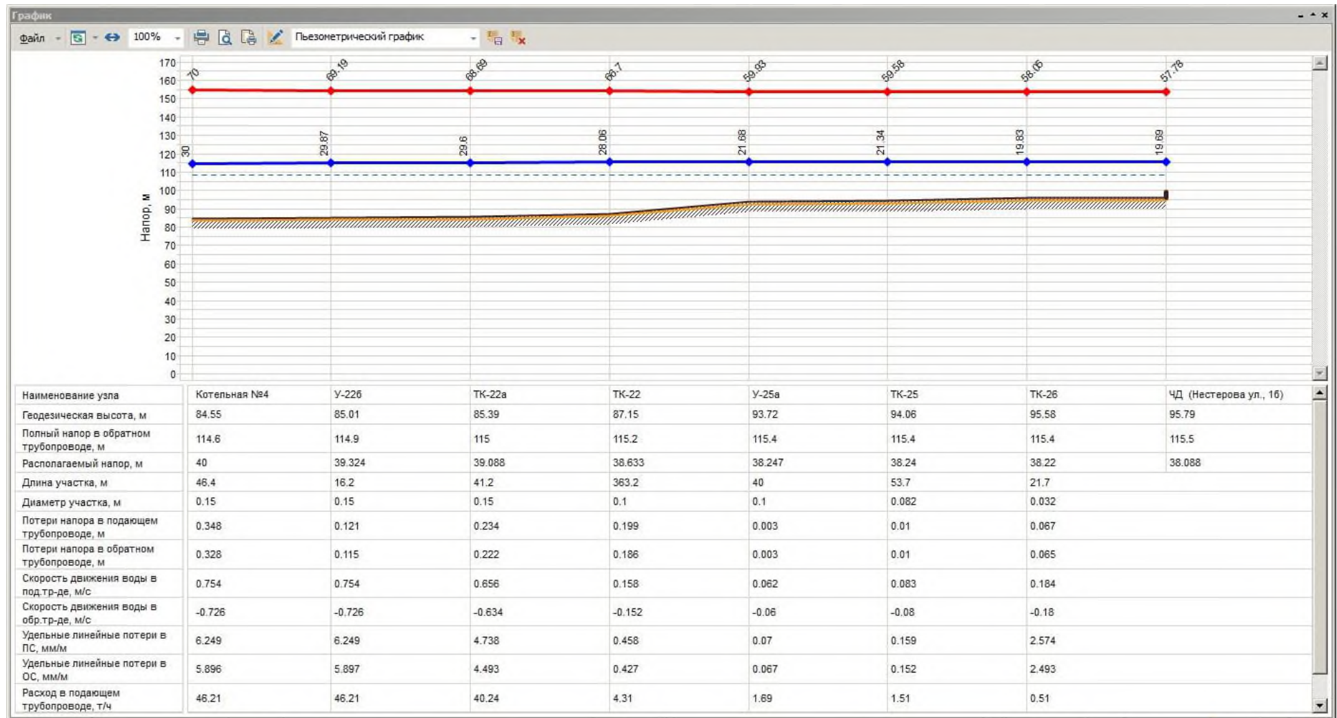
Рисунок 3.9-10 –Пьезометрический график участка №1 котельной №4 до ТК-26
