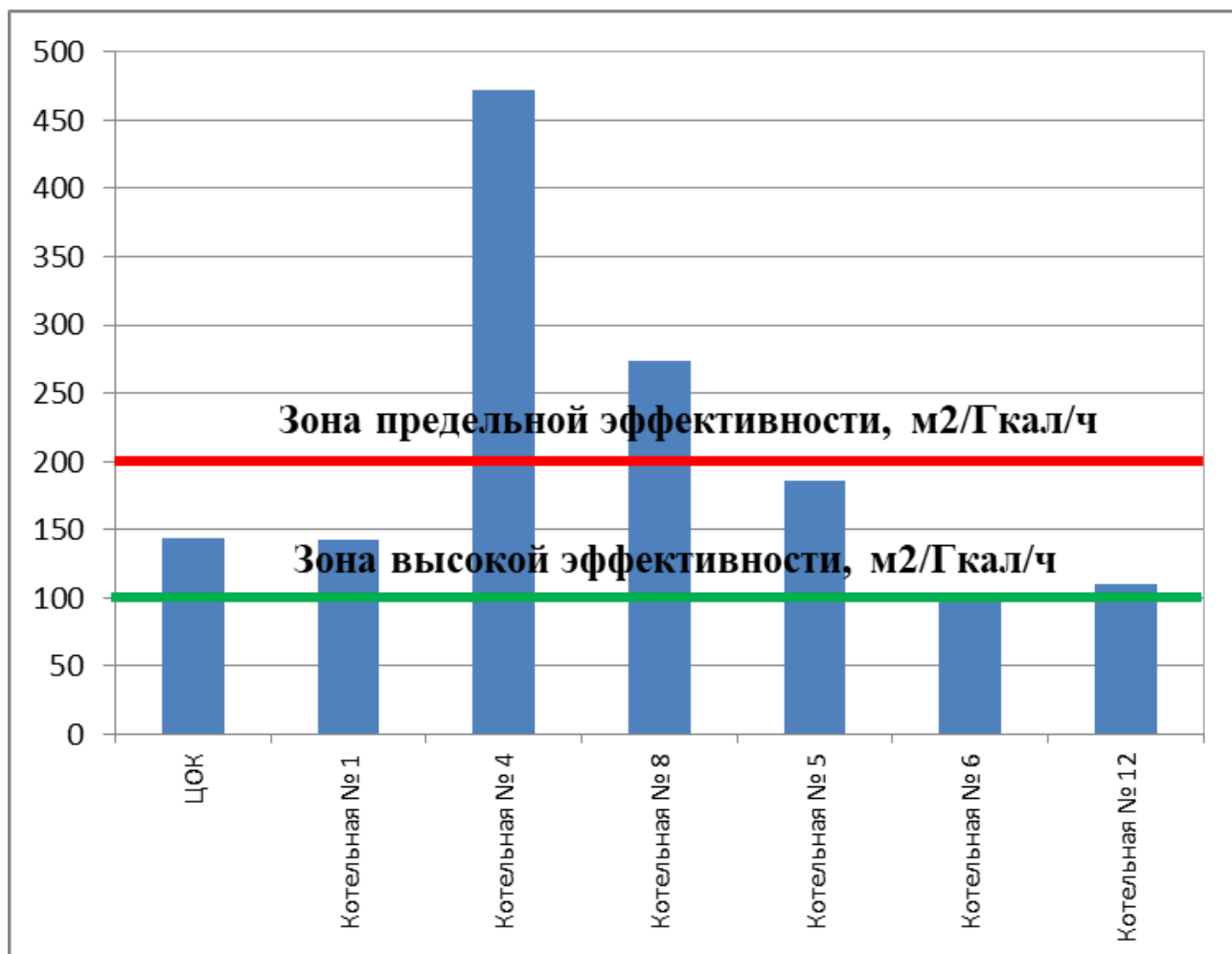
Рисунок 3.3-1 – Удельная материальная характеристика, \text{m}^2/\text{Гкал}/\text{ч}
